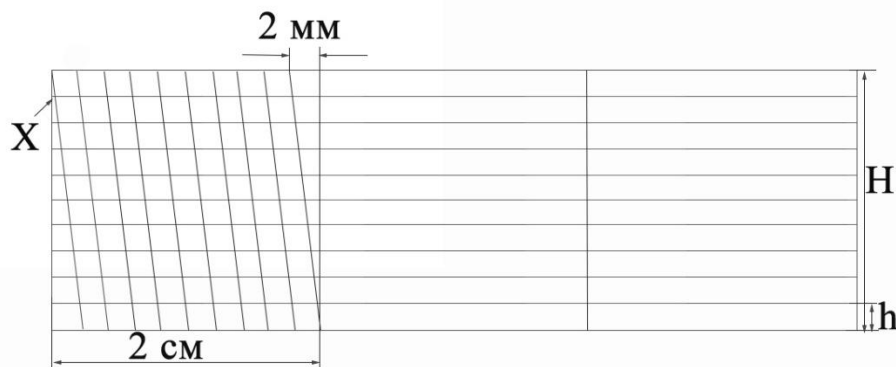
Рисунок 3 – Организация поперечного масштаба
