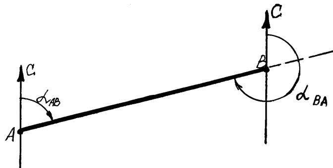
Рисунок 9 – Схема зависимости между прямыми и обратными дирекционными углами
