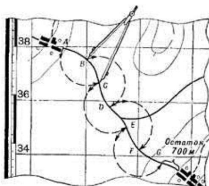
Измерение циркулем-измерителем
