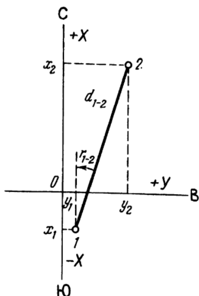
Рисунок 28 – Схема решения обратной геодезической задачи
