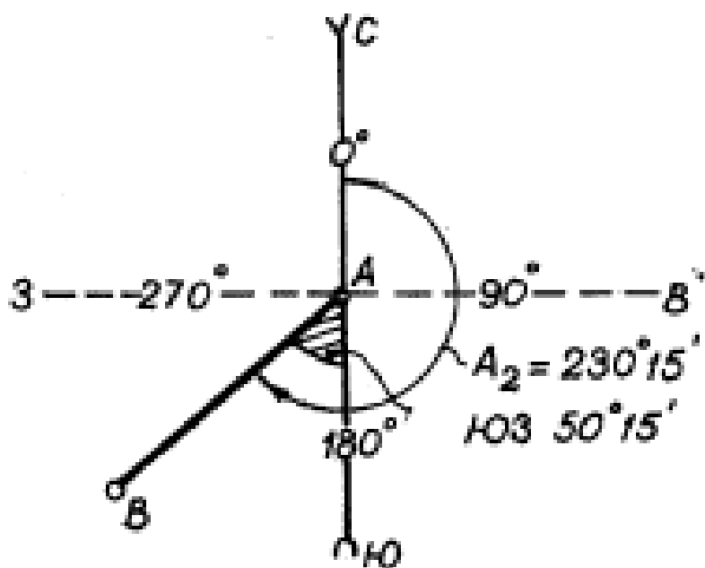
Рисунок 16 – Определение румба юго-западного направления.
