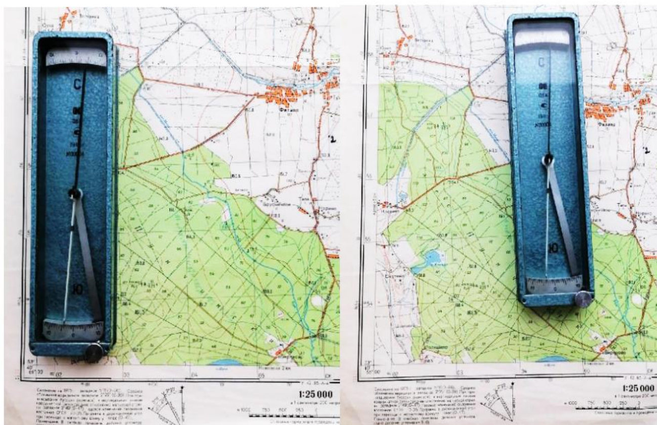
Рисунок 13 – Ориентирование карты с помощью bussоли:
