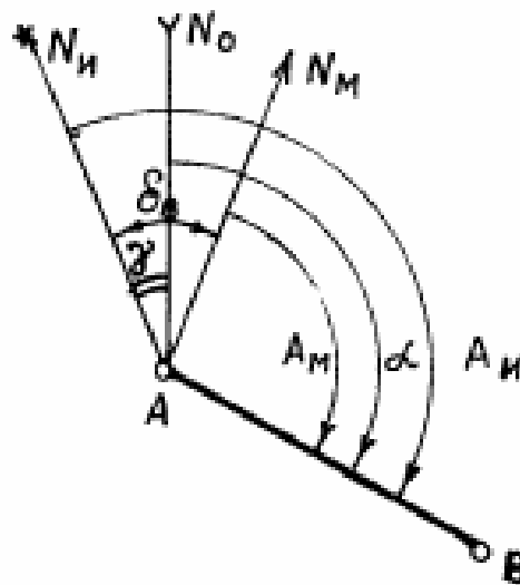
Рисунок 22 – Схема расположения направлений меридианов и углов между ними и заданным направлением AB
