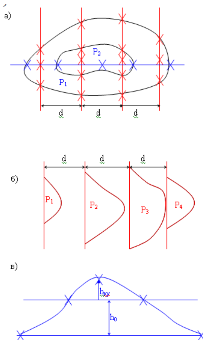
Рисунок 40 – Определение объема тел: а – план с горизонталями; б – способ вертикальных сечений; в – способ горизонтальных сечений
