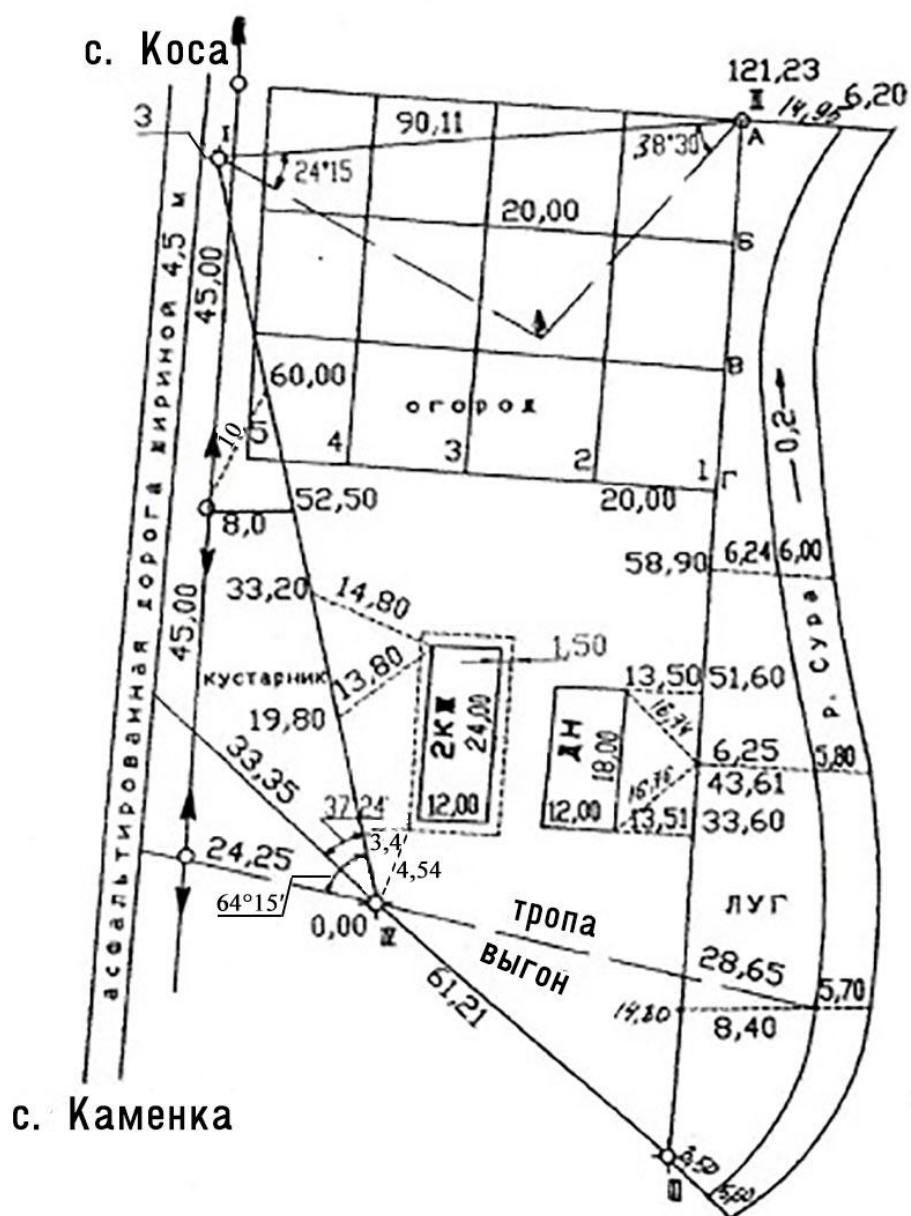
Рисунок 50 – Абрис участка землепользования
