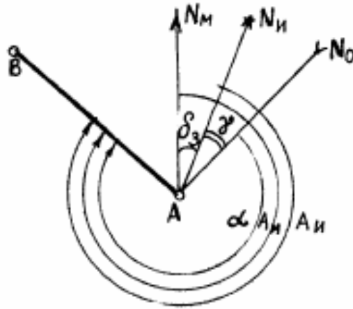
Рисунок 21 – Схема расположения направлений меридианов и углов между ними и заданным направлением AB
