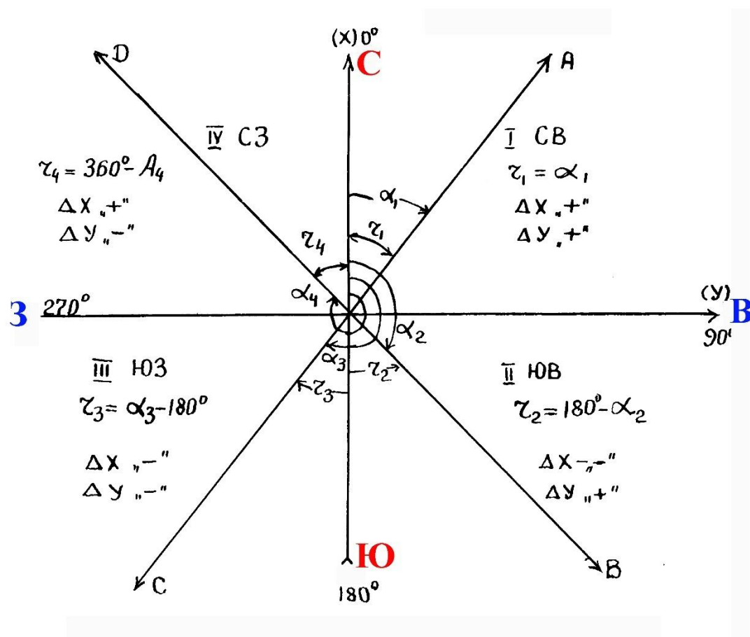
Рисунок 8 – Схема зависимости между дирекционными углами и румбами
