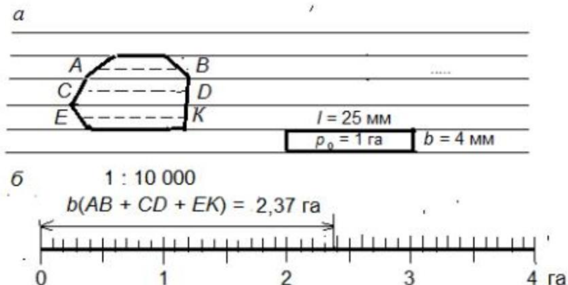
Рисунок 36 – Палетка из параллельных линий и определение площади контура по плану: а – параллельные линии палетки и контур; б – шкала площадей для плана масштаба 1: M = 1:10\,000
