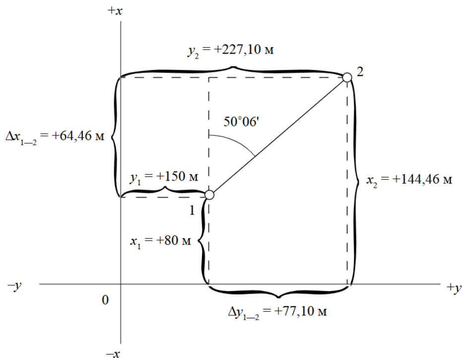
Рисунок 27 – Пример графического решения прямой геодезической задачи
