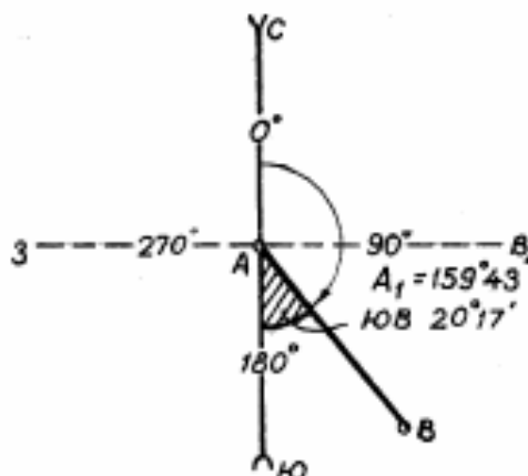
Рисунок 14 – Определение румба юго–восточного направления
