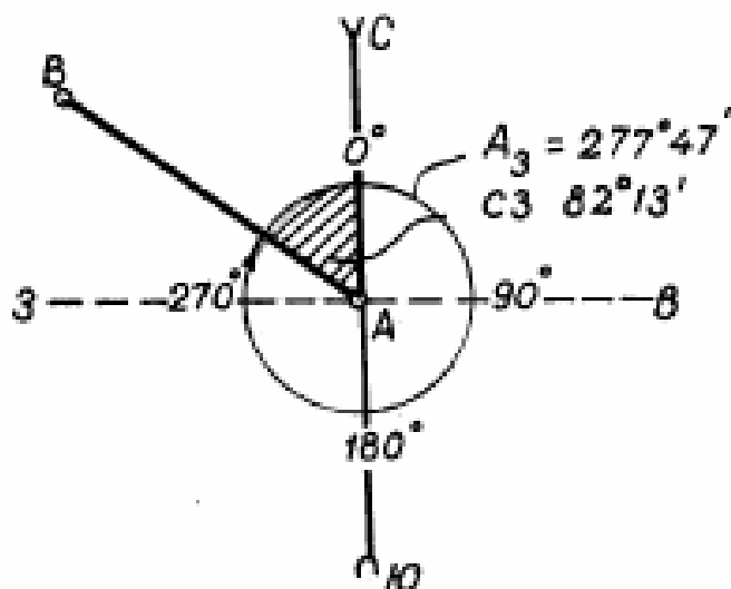
Рисунок 15 – Определение румба северо-западного направления
