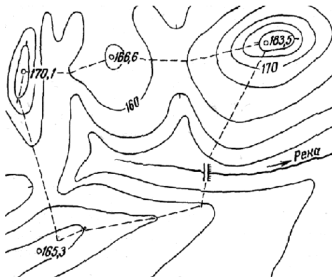
Рисунок 33 – Определение границ и площади бассейна водотока
