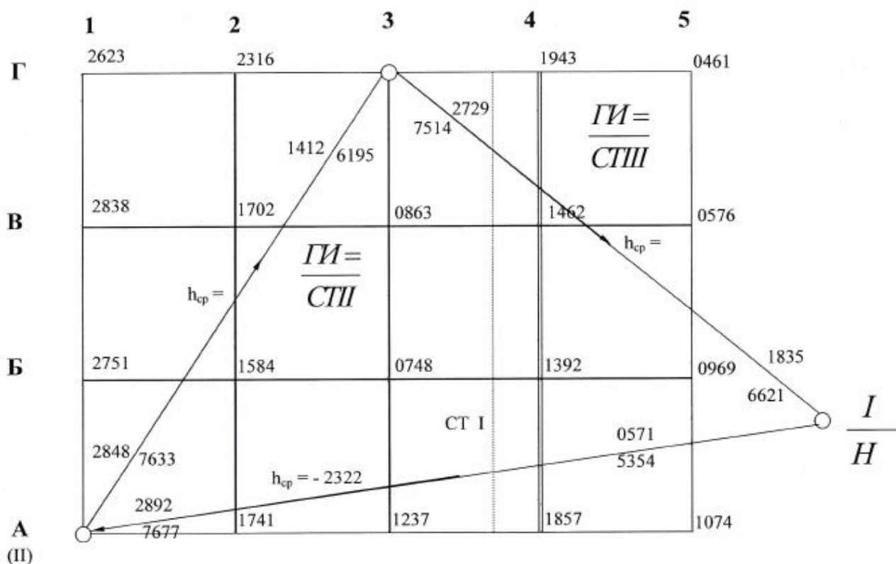
Рисунок 54 – Схема нивелирования по квадратам и его результаты
