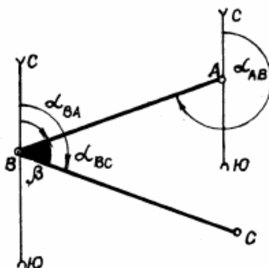
Рисунок 19 – Схема расположения угла, заключенного между тремя точками
