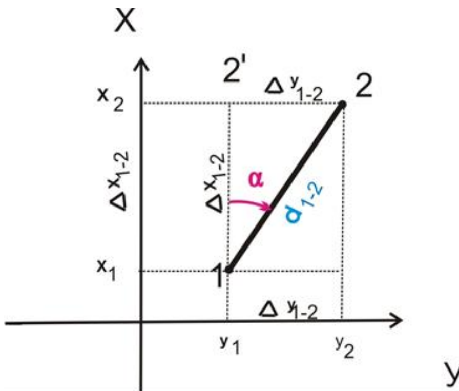
Рисунок 26 – Графическое решение прямой геодезической задачи
