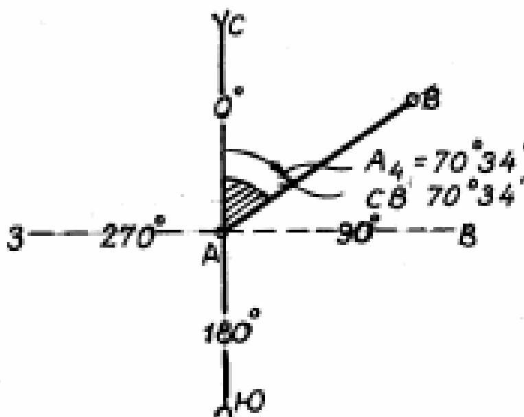
Рисунок 17 – Определение румба северо-восточного направления
