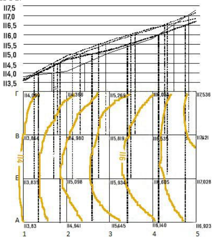
Рисунок 56 – Построение горизонталей графическим способом
