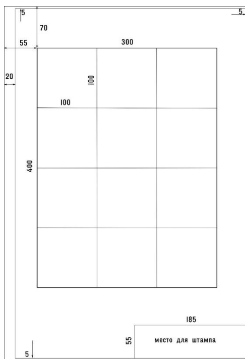
Рисунок 46 – Расположение сетки квадратов и отступы для листа A2 книжной ориентации
