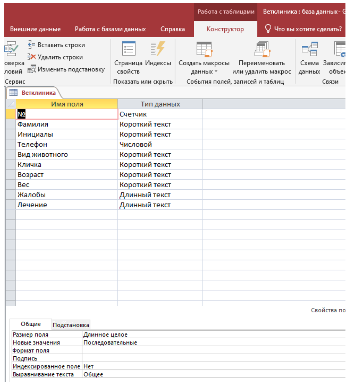
Рисунок 1. Структура БД
