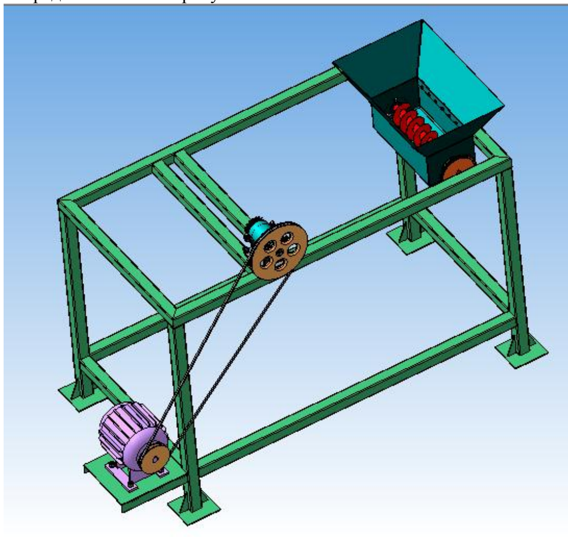
Рисунок – Лабораторная установка
