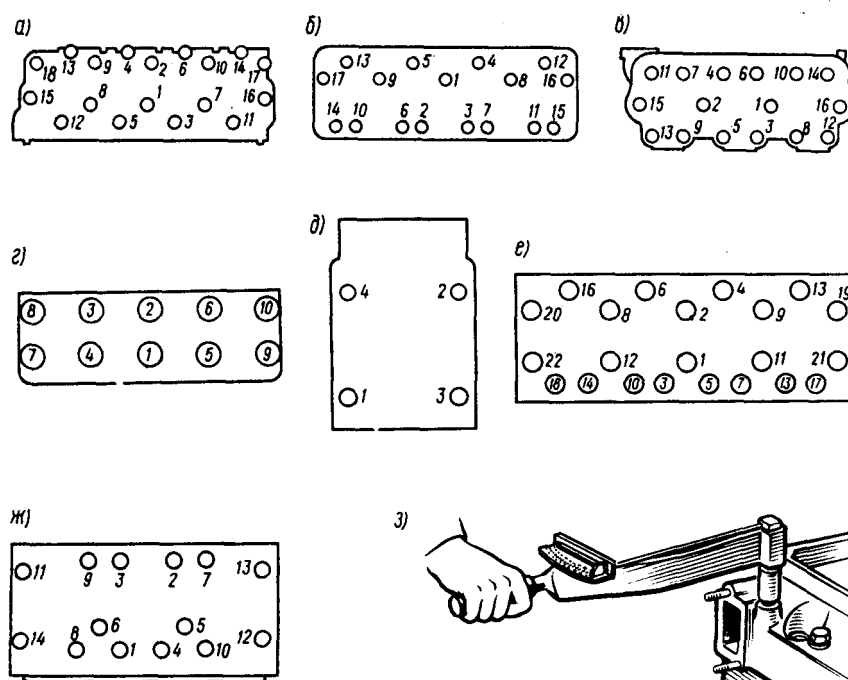
Рис. 2.1. Порядок затяжки болтов (гаек) крепления головки блока цилиндров двигателями автомобилей:
