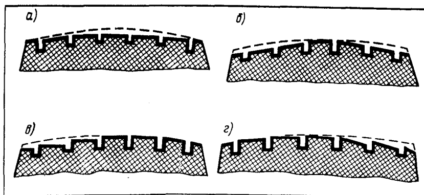
Рис. 7.1. Примеры неравномерного износа протектора вследствие неправильной эксплуатации шин или неисправностей автомобиля
