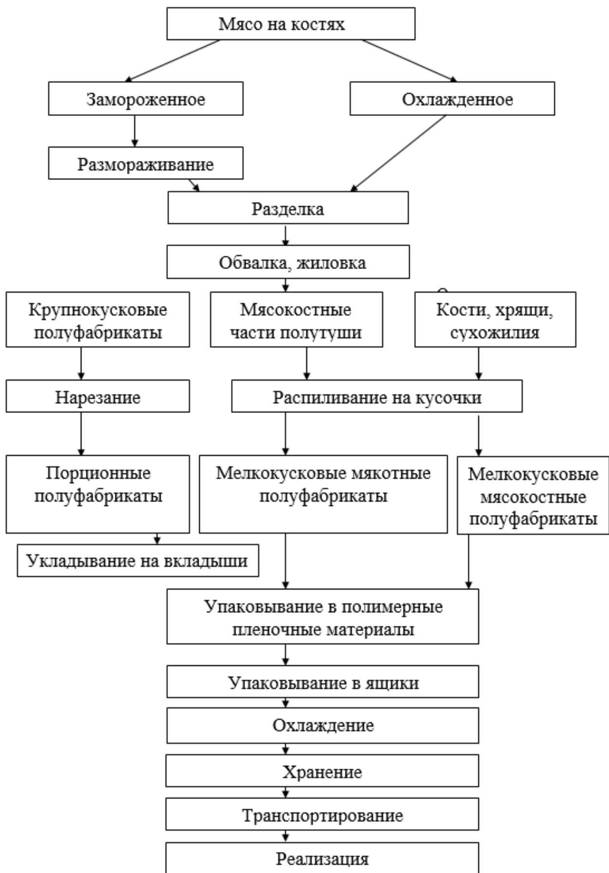
Рисунок 47 – Технологическая схема производства порционных и мелкокусковых мясных полуфабрикатов
