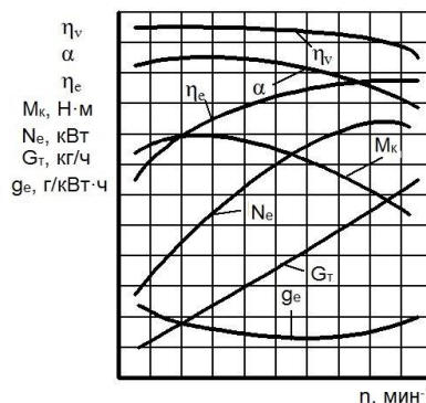
Рисунок 2 – Скоростная характеристика двигателя
