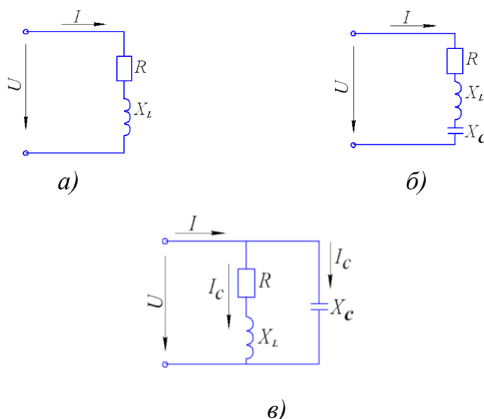
Рисунок 5.3.1 – Схемы электрических цепей к задаче 1
