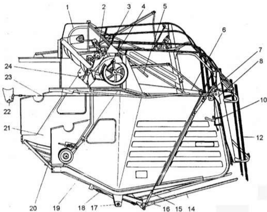
Рис. 10.1. Копнитель: 1-капот; 2-соломонабиватель; 3-механизм сбрасывания копны; 4-гидроцилиндр открытия копнителя; 5-сигнализатор; 6-тяга механизма сбрасывания; 7-гидроцилиндр закрытия копнителя; 8-клапан копнителя; 9-поперечина клапана верхняя; 10-сигнализатор открытия копнителя; 12-планка вертикальная; 14-палец днища; 15-гайка стяжная; 16-звено пальца днища промежуточное; 17-ось крепления днища; 18-пружина днища; 19-боковина левая; 20-днище; 21-боковина правая; 22-гидрораспределитель копнителя; 23-тяга гидрораспределителя; 24-щиток сброса соломы
