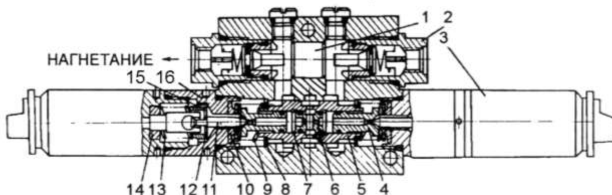
Рис. 14.5. Рабочая секция (нейтральное положение; напряжение отсутствует): 1- поршень; 2-клапан запорный; 3-клапан электромагнитный; 4-седло; 5-золотник; 6, 15-втулки; 7- кольцо; 8, 10, 12-шайбы; 9, 13-пружины; 11-игла; 14-якорь; 16- проставка
