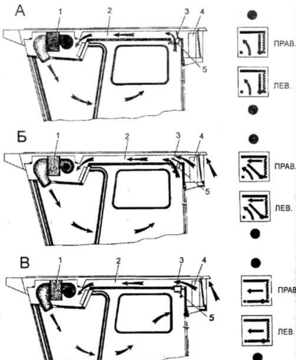
Рис. 19.3. Система циркуляции воздуха в кабине комбайна: 1-кондиционер; 2- канал подачи воздуха; 3-клапан рециркуляционный; 4-фильтр; 5-фильтр рециркуляционного клапана; А-режим кондиционирования с рецеркуляцией; Б-режим рециркуляции с забором свежего воздуха в пропорции 50/50; В-режим вентиляции с забором 100% свежего воздуха через фильтр
