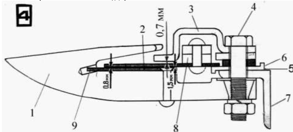
Рис. 2.14. Схема режущего аппарата: а - среднее положение рычага; б - крайнее положение рычага; 1 - палец; 2 - сегмент; 3 - прижим; 4 - болт; 5 - регулировочная прокладка; 6 - пластина трения; 7 - уголок; 8 - спинка ножа; 9 - вкладыш
