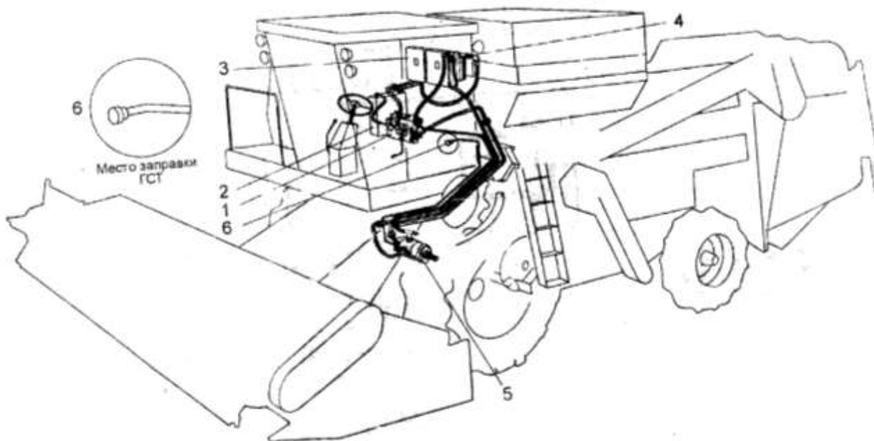
Рис. 14.3. Схема гидропривода ходовой части: 1-аксиально-поршневой насос НП-90; 2-радиатор масляный 100У-08.003; 3-бак РСМ-10.09.09.080В; 4-фильтр всасывающий ФВ-10.00.000 или ФС 32АВЗ0П10Н1; 5-аксиально-поршневой гидромотор МП-90Б; 6-полумуфта наружная Н.036.67.100-10
