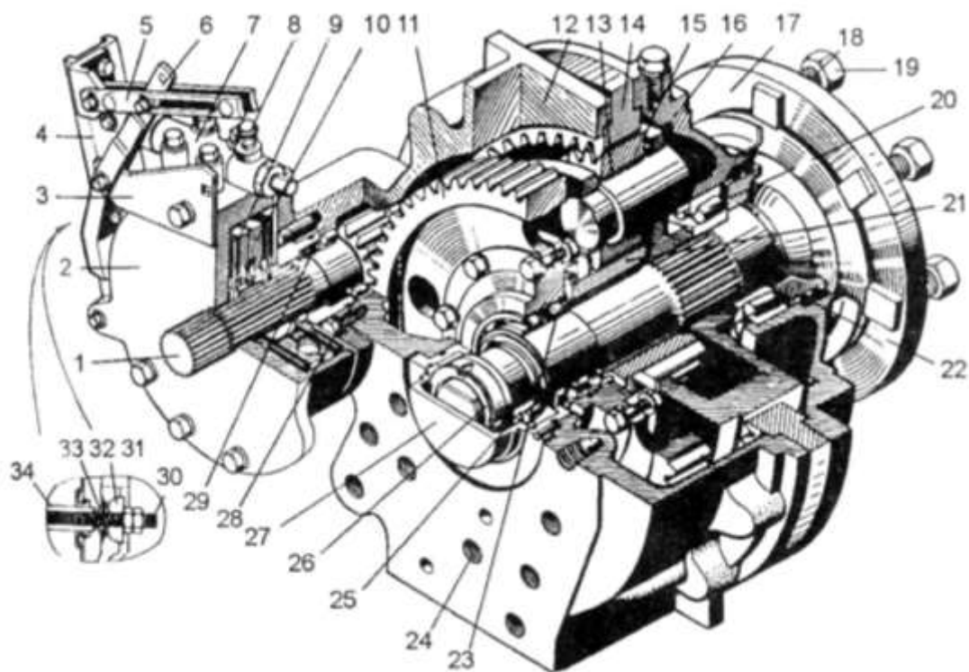
Рис. 13.2. Бортовой редуктор: 1-вал-шестерня; 2-корпус тормоза, 3-кронштейн стояночного тормоза; 4-рычаг гидроцилиндра; 5-рычаг стояночного тормоза; 6-рычаг управления стояночным тормозом; 7-гидроцилиндр тормоза; 8-штуцер прокачки; 9-диск тормоза фрикционный; 10-диск тормоза; 11-колесо зубчатое; 12-корпус; 13-подшипник игольчатый 664913Д; 14-шестерня эпициклическая; 15-шестерня-сателлит; 16-крышка корпуса; 17-ось ведущего колеса; 18-болт крепления колеса; 19-гайка крепления колеса; 20-подшипник роликовый 7519; 21-шестерня солнечная; 22, 29-манжеты; 23-шарикоподшипник 215; 24- отверстие крепления редуктора к балке моста; 25-подшипник роликовый 7513; 26, 31-гайки; 27-крышки; 28-подшипник роликовый 42211; 30-болт установочный; 32-прокладка сферическая; 33-пружина; 34-вилка тормозная
