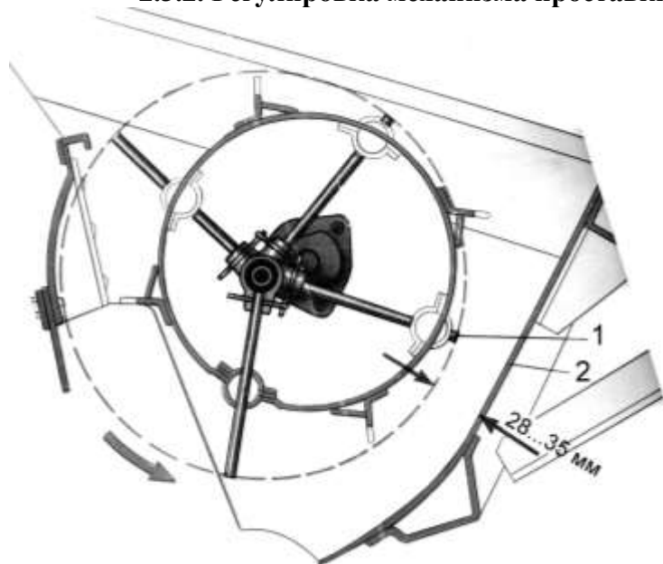
Рис. 2.20. Схема пальчикового механизма проставки: 1-палец; 2-днище
