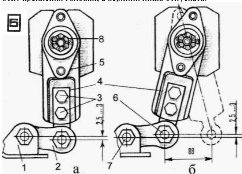
Рис.2.15. Схема регулировки привода ножа: 1 – головка ножа; 2 – щетка; 3 – болты; 4 – головка рычага; 5 – рычаг; 6 – ось шарнира головки рычага; 7 – ось шарнира головки ножа; 8-гайка
