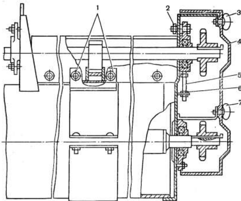
Рис. 7.3. Регулировка привода выгрузного наклонного шнека: 1, 2, 3, 7 - болты; 4- кожух; 5 - тяга;
