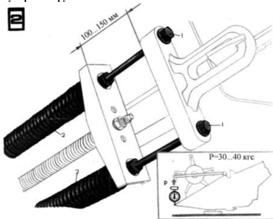
Рис.2.3. Схема пружинных блоков: 1 – болты регулировочные; 2 – пружинные блоки
