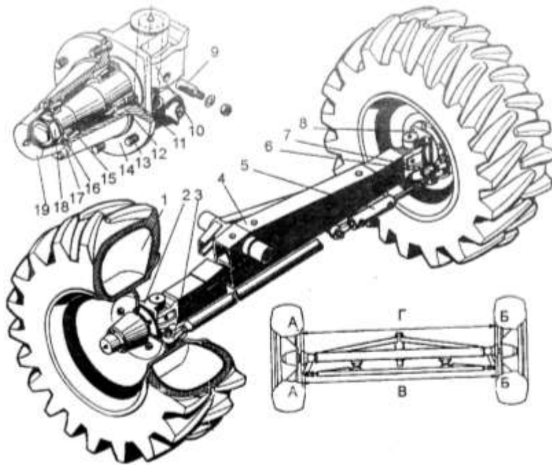
Рис. 11.1. Мост управляемых колес: 1 - колесо управляемое; 2, 8 - кулаки поворотные левый и правый; 3, 7 - рычаги рулевой трапеции; 4 - балка моста; 5 - гидроцилиндры поворота; 6-тяги рулевая; 9 - клин шкворня; 10 - шкворень; 11 - сальник; 12 - подшипник 7613А; 13 - болты крепления колеса; 14 - ступица; 15-подшипник 7610А; 16 - втулка; 17 - шайба; 18 - гайка; 19-колпак ступицы; А, Б - точки замера сходимости колес; В, Г -
