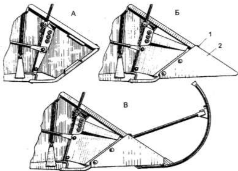
Рис. 2.22. Делители: А - боковина жатки, выполняющая роль делителя; Б - боковина жатки с носком; В - прутковый делитель; 1 - болт крепления носка; 2 - носок
