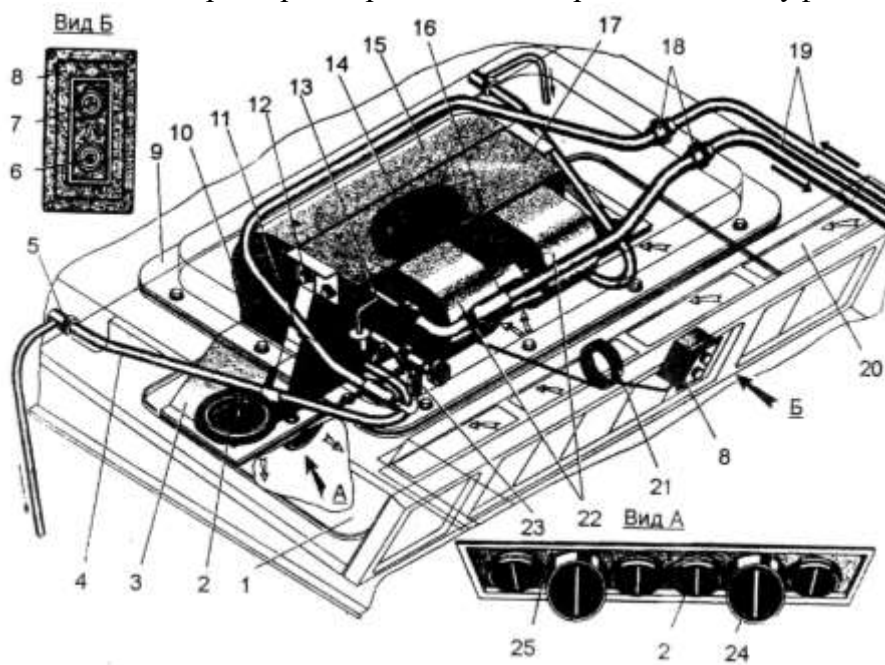
Рис. 19.1. Установка в кабине испарителя кондиционера «Конвекта»: 1-воздушный отсек; 2-дефлектор; 3-воздуховод; 4-трубка слива конденсата; 5-штуцер; 6-рукоятка включения компрессора и управления термостатом; 7-рукоятка включения и регулировки оборотов вентиляторов; 8-панель управления; 9-люк верхней кабины; 10-уплотнение; 11-кронштейн; 12-болт; 13, 23-патрубки отвода и подвода фреона; 14-испаритель; 15-дефлектор; 16- электродвигатель; 17-испарительно-вентиляционный блок; 18-втулки уплотняющие; 19-рукава; 20-отверстия подвода воздуха в воздушном отсеке; 21-трубка термостата; 22-вентиляторы; 24-патрубки поворотные с дефлекторами; 25-панель дефлекторов
