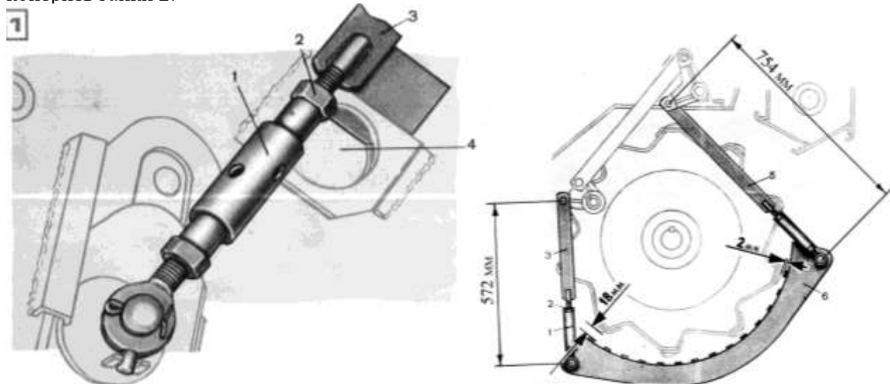
Рис. 5.2. Схема регулировки положения подбарабанья: 1,2 - гайки стяжные; 3 - передние тяги; 4 - смотровые окна; 5 - задние тяги; 6 - подбарабанье
