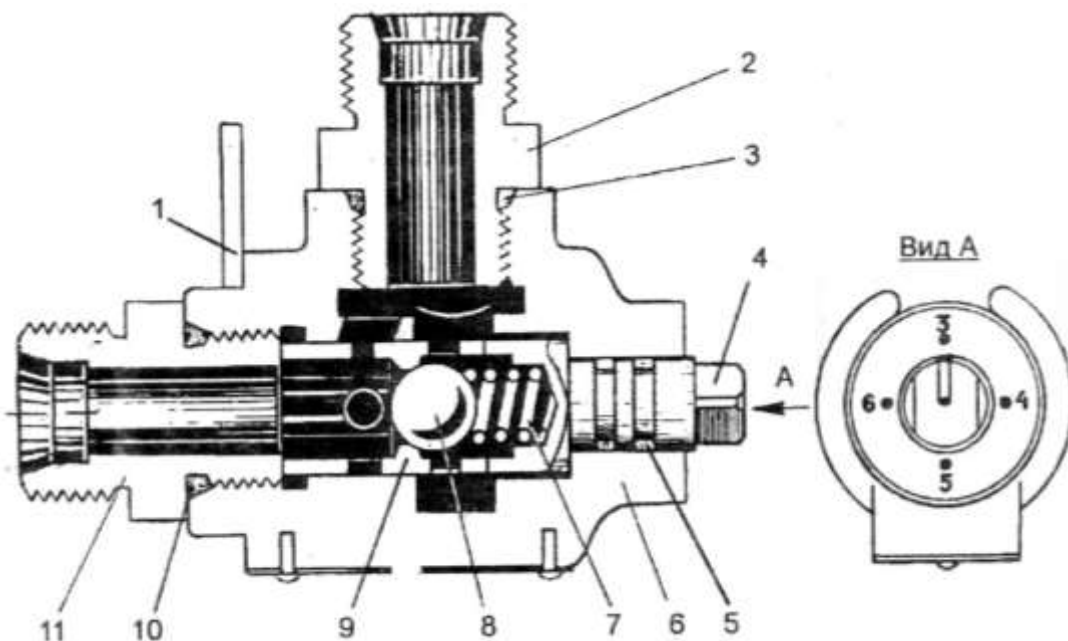
Рис. 14.9. Клапан дросселирующий настраиваемый КДН 00.000-06: 1-кронштейн; 2, 11-штуцеры; 3, 5, 10-кольца уплотнительные; 4-шпindel; 6-корпус; 7-пружина; 8-шарик; 9-золотник дроссельный
