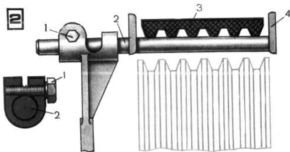
Рис. 5.5. Схема регулировки положения пальца подъемника: 1 - болт стяжной; 2 - палец; 3 - ремень; 4 - направляющие щечки
