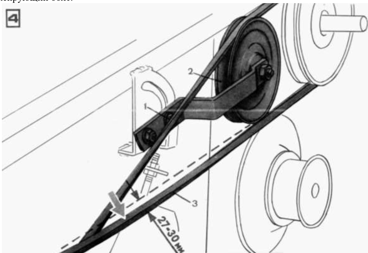
Рис. 4.5. Схема регулировки натяжения приводного ремня: 1 - болт фиксирующий; 2 - натяжной ролик; 3 - ремень
