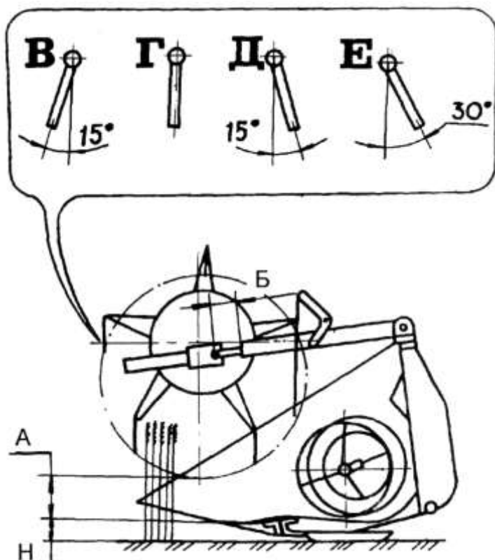
Рис. 2.10. Схема установки мотовила: А-по высоте; Б-по горизонтали; Н-высота среза стеблей; Б, Г, Д, Е – наклон граблин
