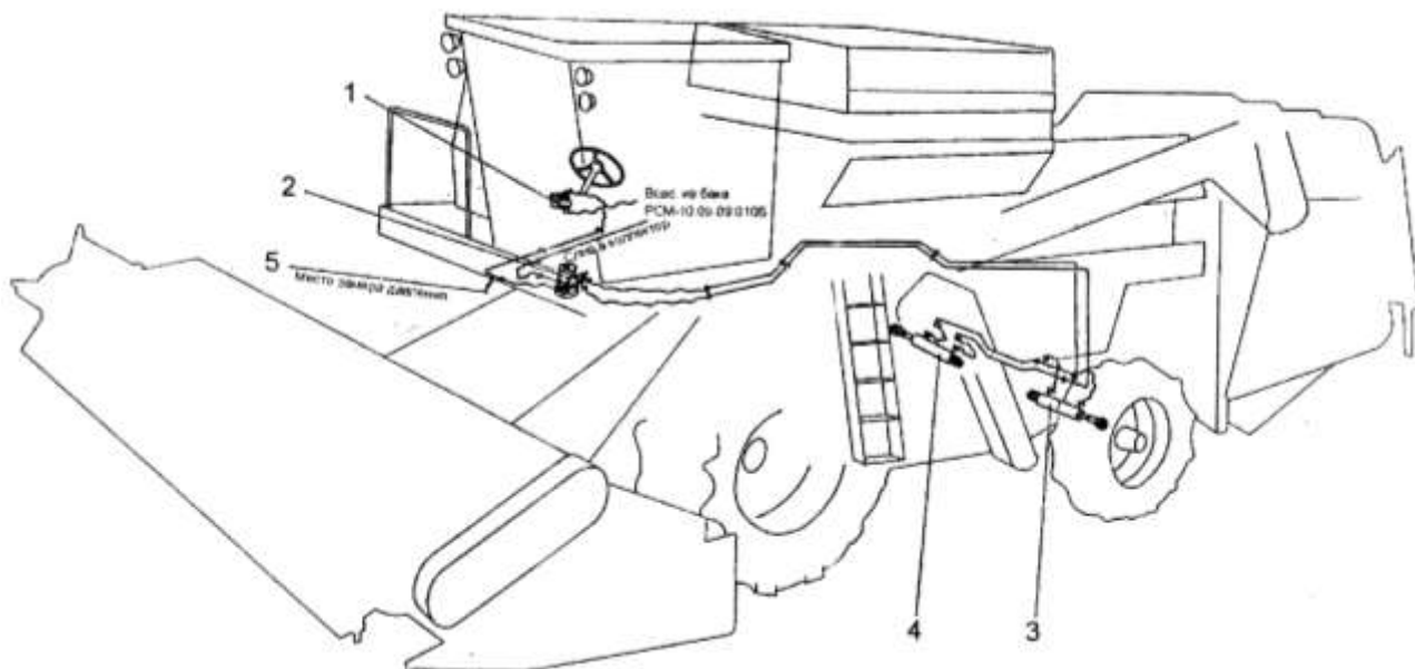
Рис. 14.2. Схема гидросистемы рулевого управления: 1-насос НШ-ЮВ-3-Л (двигатель СМД и Д461-51) или НШ-10Г-3-Л (двигатели ЯМЗ и КАМАЗ); 2-агрегат рулевой АР-125-16; 3, 4- гидроцилиндры управляемых колес ГЦ 50.200.16.000А-01; 5-муфта Н036.67. ЮО-10
