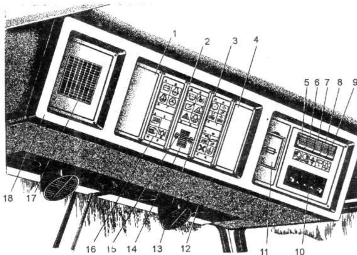
Рис. 15.4. Верхняя панель приборов (см. рис.15.1): 1, 4-заглушки; 2 -блок А10 световой и звуковой сигнализации (БЗС); 3-блок А11 световой сигнализации (БСС); 5-включение рабочих фар; 6-включение фары выгрузного шнека; 7-включение компрессора кондиционера или вентилятора кабины (при оборудовании кабины вентиляторами); 8-включение стеклоочистителя; 9-включение фары-мигалки; 10-заглушка; 11-блок предохранителей; 12- панель системы кондиционирования или вентиляции; 13-регулятор громкости; 14-зуммер; 15- контроль ламп табло; 16- блок А9 световой сигнализации (БСС); 17-заглушка, 18- фальшпанель; А-зарядка аккумуляторов; Б-давление масла в двигателе ниже нормы; В- температура воды двигателя выше нормы; Д-забивание, пространства над соломотрясом; Ж-заполнен копнитель; З-забивание пневмоэлеватора; И-заполнение бункера; К- стояночный тормоз включен; Л-клапан копнителя открыт; М-потери выше нормы; Н-забивание фильтра основной гидросистемы; П-обороты молотильного барабана ниже нормы; Р- обороты вала очистки ниже нормы; С-обороты колосового шнека ниже нормы; Т - обороты зернового шнека ниже нормы; У-обороты соломонабивателя ниже нормы - забивание шнека половой; Ф- обороты вала соломотряса ниже нормы; Х-забивание барабана измельчителя; Ц-забивание вентилятора измельчителя
