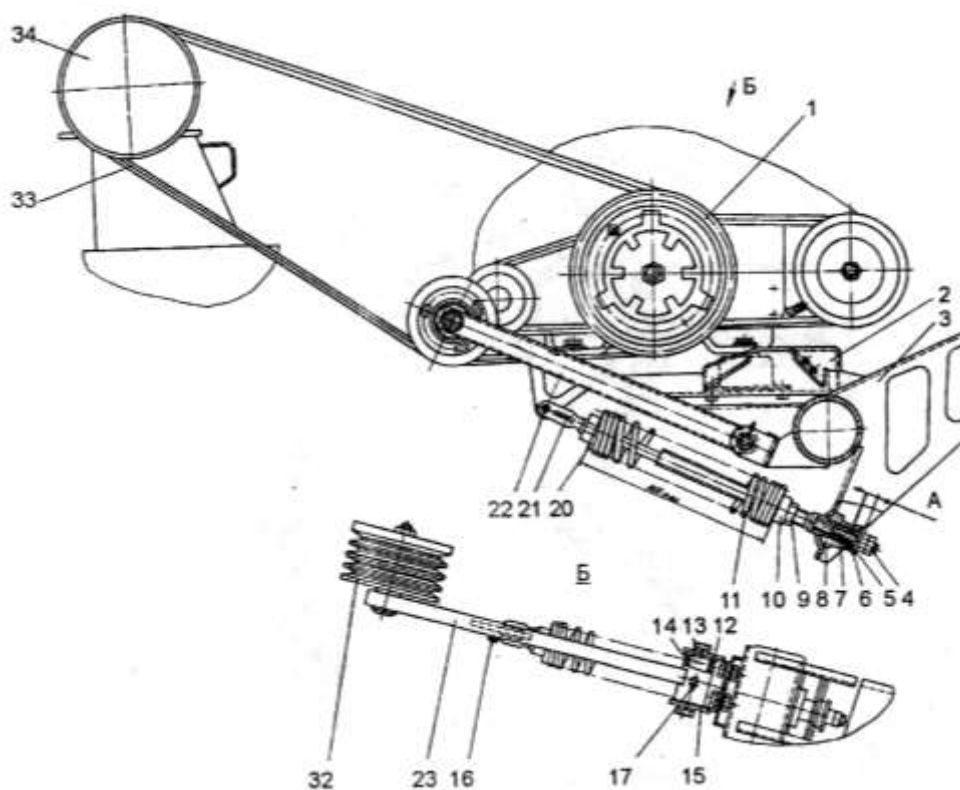
Рис. 14.11. Привод гидронасоса ходовой части комбайна «Дон-1500Б»: 1-шків двигателя; 2-рама моторно-силовой установки; 3-кронштейн рамы; 4, 9-гайки; 5-шайба; 6- амортизатор; 7-шпилька; 8-втулка натяжная; 10, 20-пробки; 11-пружина; 12, 14-шайбы; 13-втулки; 15- кольцо стопорное; 16-масленка; 17, 22-оси; 21- вилка; 23-рычаг шкива; 32-шків натяжной; 33-ремень приводной; 34-шків привода гидронасоса; А-толщина амортизатора 6, равная 13...15 мм
