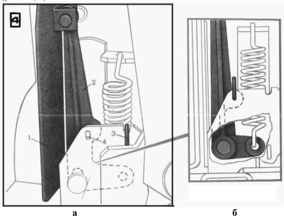
Рис. 2.5. Схема боковых щитков: а-щиток прижат; б-щиток отведён; 1-щиток; 2-рычаг; 3-шплинт; 4-отверстие
