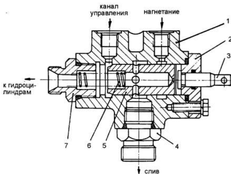
Рис. 14.10. Распределитель копнителя: 1-корпус; 2-крышка; 3-толкатель; 4, 7-штуцеры; 5-золотник; 6-пружина.
