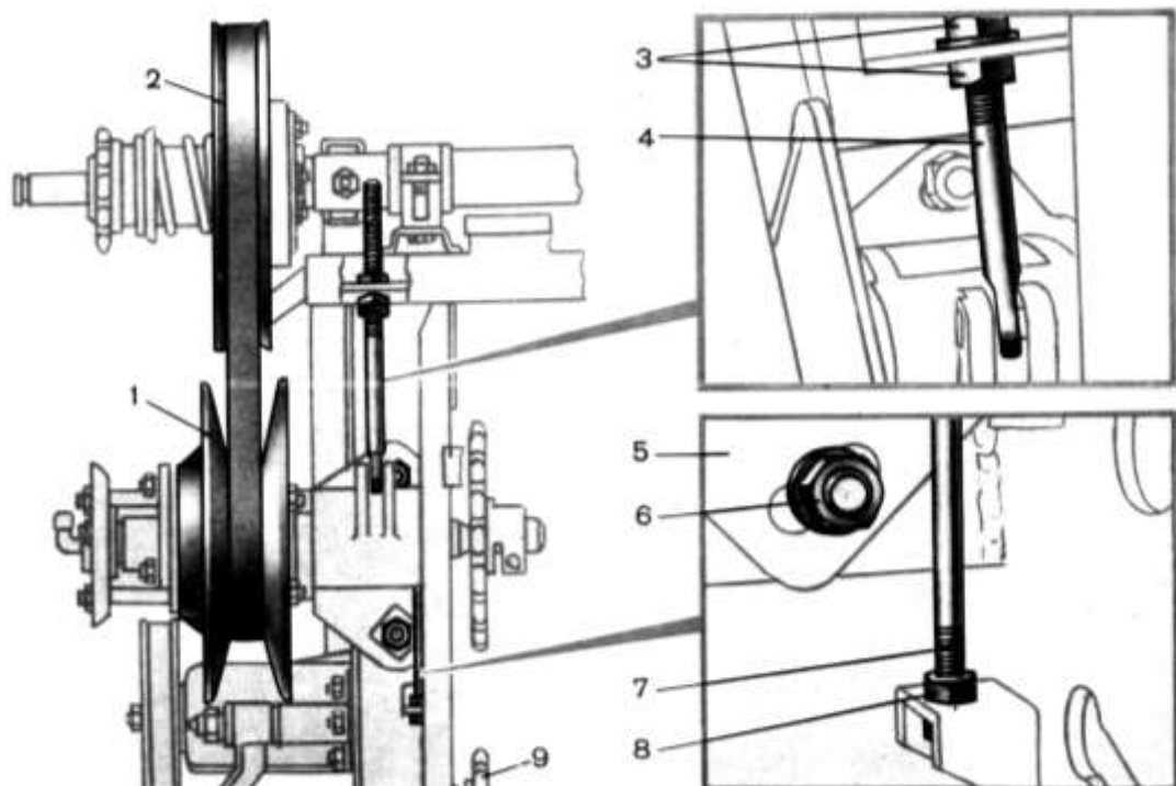
Рис. 2.11. Вариатор жатки: 1-шкив ведущий; 2-шкив ведомый; 3,8-гайки; 4,7-винты; 5-плита; 6-болт; 9-звёздочка.
