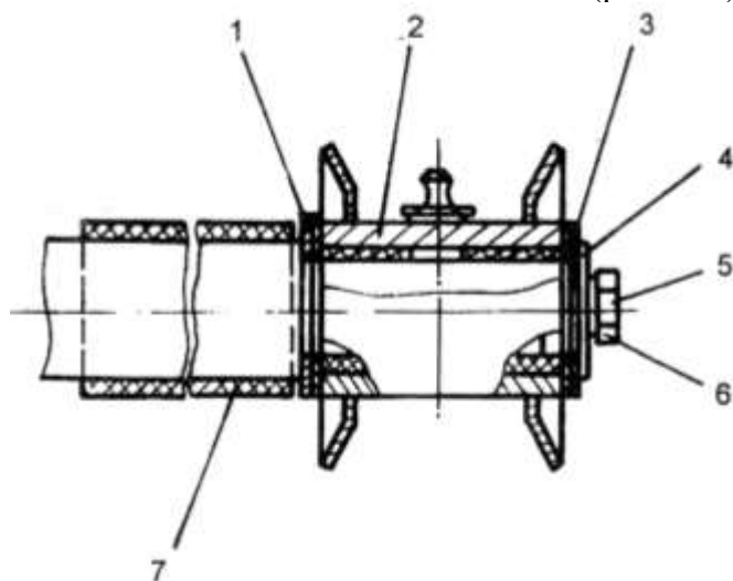
Рис. 2.12. Правый подшипник мотовила: 1, 3-пакеты регулировочных шайб; 2-подшипник; 4-шайба специальная; 5-болт с левой резьбой; 6-шайба; 7-кожух защитный.
