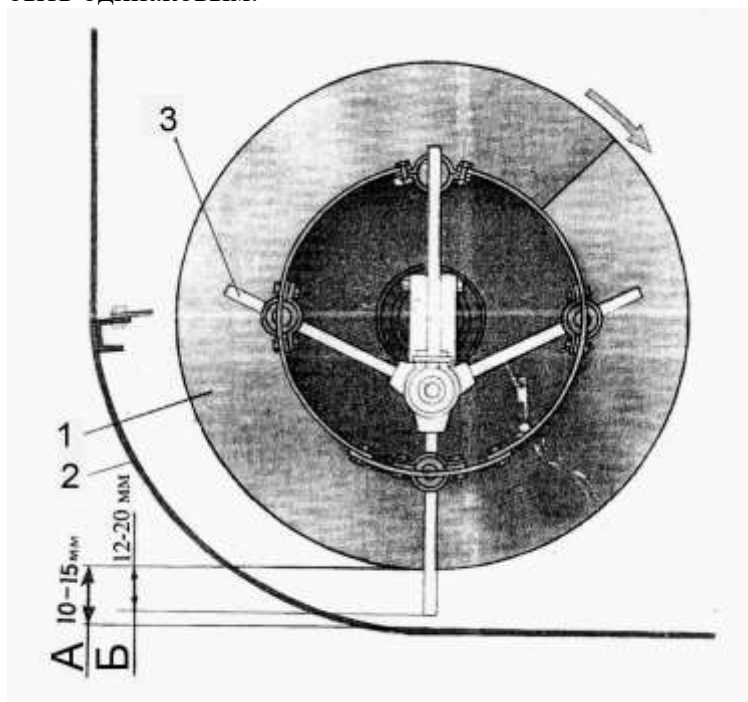
Рис. 2.18. Схема шнека: 1-спираль шнека; 2-днище; 3-палец шнека
