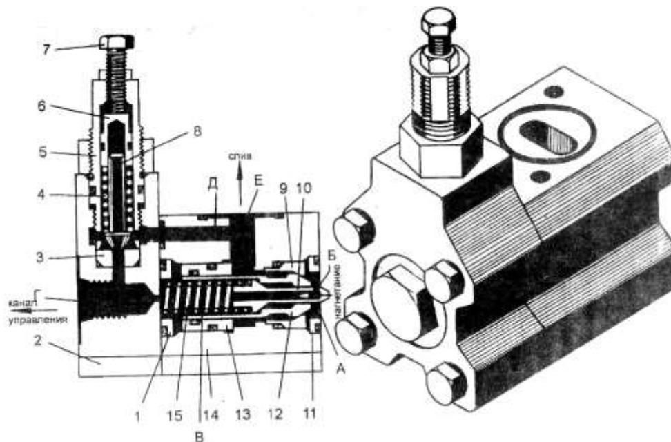
Рис. 14.7. Клапан напорный КН 50.12,5 или 108.00.000В: 1, 11-шайбы; 2-крышка; 3, 9-седла; 4, 15-пружины; 5, 13-втулки; 6-поршень; 7-болт; 8-запорный элемент; 10-клапан; 12-клапан; 14-корпус; А-полость нагнетания; Б-дроссельное отверстие; В-полость внутренняя; Г-полость выхода потока; Д-полость сливная предохранительного клапана; Е-полость слива
