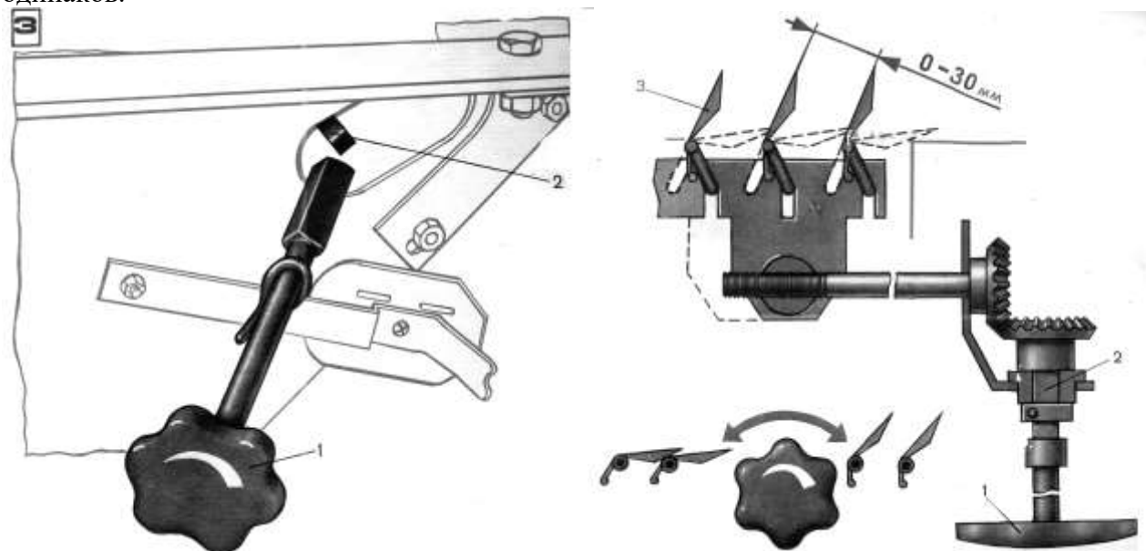
Рис.6.4. Схема регулировки наклона жалюзи решёт: 1-маховик; 2-вал; 3-решёта
