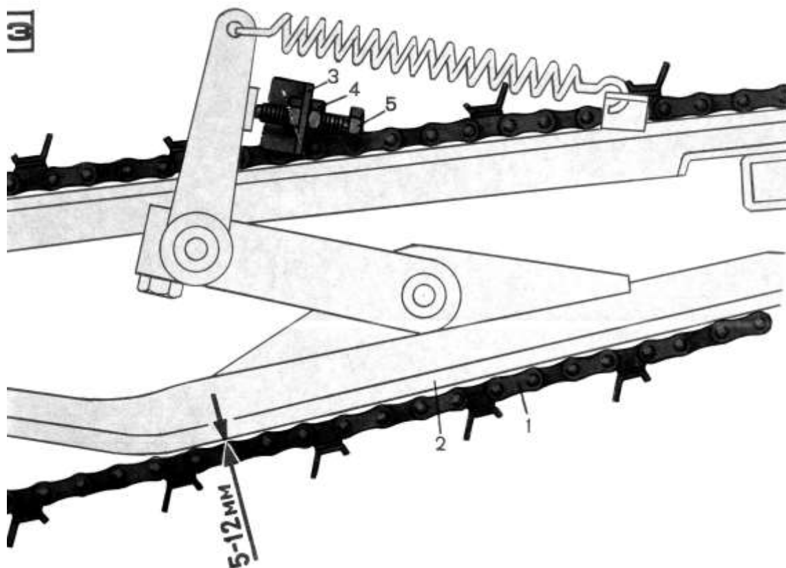
Рис. 3.4. Схема регулировки положения ползьев: 1 – цепь; 2 – ползья; 3 – кронштейн; 4 – контргайка; 5 – болт
