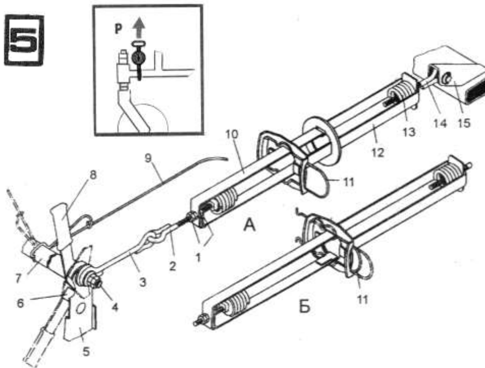
Рис. 4.6. Разгружающее устройство: А - установка разгружающего устройства; Б - транспортное положение фиксатора (рабочее его положение изображено штрихпунктирными линиями); 1 - гайка регулировочная; 2 - растяжка; 3 - шпренгель; 4 - цапфа эксцентриковая; 5 - стойка; 6 - упор; 7 - балка нормализатора; 8 - рычаг; 9 - палец; 10, 12 - обоймы; 11 - фиксатор; 13 - пружина растяжения; 14 - растяжка; 15 - балка платформы
