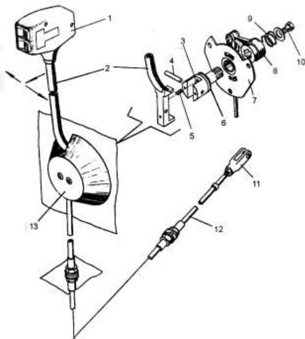
Рис. 11.4. Механизм управления гидростатическим приводом хода: 1-рукоятка управления ГСТ с клавишами подъема и опускания жатки и мотовила и звукового сигнала; 2-рычаг; 3-вал; 4-штифт; 5-пружина; 6-фрикционная шайба; 7-диск; 8-рычаг; 9-пружина; 10- регулировочный болт; 11-вилка; 12-трос двустороннего действия; 13-крышка
