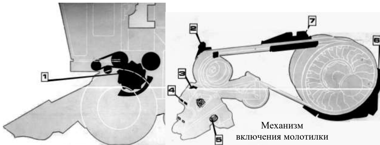
Рис. 5.1. Схема регулировки молотильного устройства и механизма включения молотилки: 1- молотильное устройство; 2-палец подъёмника; 3-подъёмник; 4-боковина кронштейна; 5-пружина; 6-нижний кожух; 7-верхний кожух.
