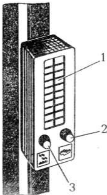
Рис. 15.6. Блок индикации потерь (БИП): 1-шкала; 2-ручка настройки канала очистки; 3-ручка настройки канала соломотряса
