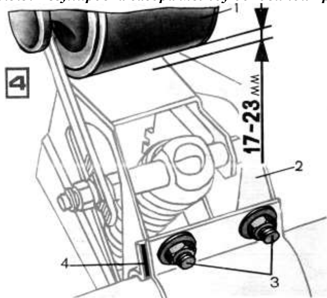
Рис. 5.7. Схема регулировки зазора между боковиной кронштейна и шкивом двигателя: 1-шкив двигателя; 2-опорный кронштейн; 3-болты; 4-регулирующие прокладки
