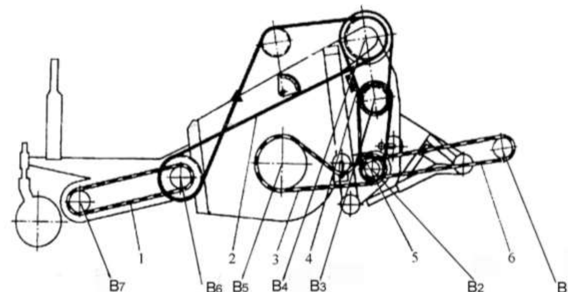
Рис.16.2. Кинематическая схема платформы-подборщика: 1-передача на ведомый вал транспортёра подборщика; 2-передача на ведущий вал подборщика; 3-передача на вал шнека; 4-передача на верхний вал вариатора; 5-передача на вал шнека; 6-передача на приводной вал; В1-вал трансмиссионный; В2-вал приводной; В3-вал нижний вариатора; В4-вал верхний вариатора; В5-вал шнека; В6-вал ведущий подборщика; В7-вал ведомый подборщика
