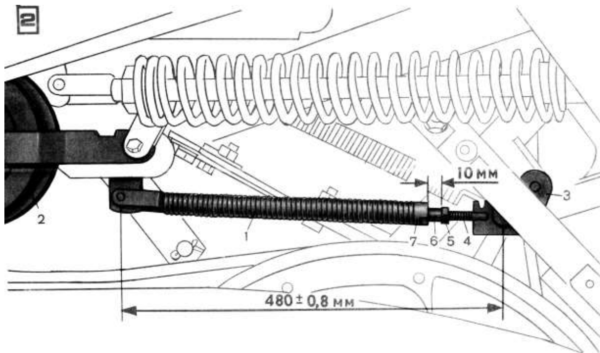
Рис. 3.3. Схема механизма включения привода: 1 – пружина; 2 – шкив; 3 – кривошип; 4 – тяга; 5 – контргайка; 6 – ось; 7 – пробка
