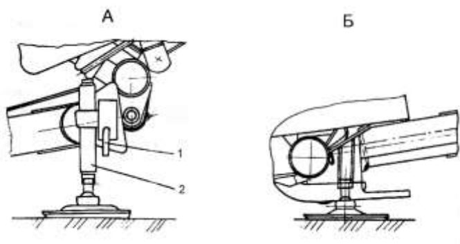
Рис. 24.1. Схема установки опор жатвенной части: А- установка опор на жатвенной части с жатками захватом 7 м; Б- установка опор на жатвенной части с жатками захватом 8,6 м; 1- опора; 2- штырь
