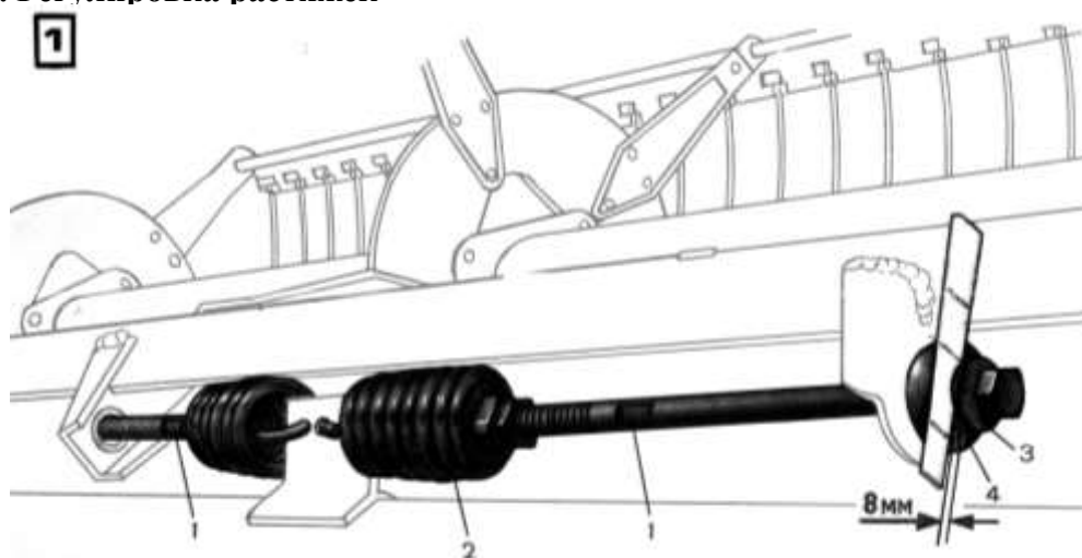
Рис. 2.2. 1 Схема растяжек: 1 – натяжные винты растяжек; 2 – пружины растяжек; 3 – головка винта; 4 – сферический подпятник
