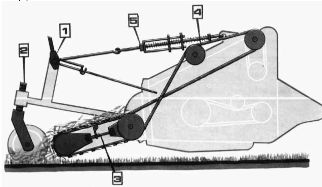
Рис. 4.1. Схема платформы-подборщика: 1-нормализатор; 2- колёса опорные; 3-винт натяжения тяговых цепей транспортёра; 4-ремень приводной; 5-разгружающее устройство
