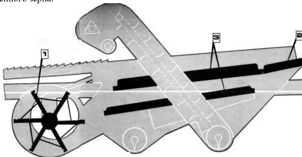
Рис.6.1. Схема регулировки очистки: 1- вентилятор; 2- удлинитель; 3-верхнее и нижнее решёта
