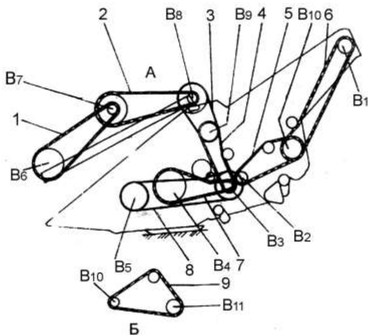
Рис. 16.1. Схема передач жаточной части: 1-передача на вал мотовила (от В7 на В6); 2- передача на вал контрпривода мотовила (от В8 на В7); 3- передача на ведомый вал вариатора мотовила (от В9 на В8); 4- передача на ведущий вал вариатора мотовила (от В3 на В9); 5-передача на контрприводной вал (от В10 на В2); 6-передача на трансмиссионный вал (от В1 на В10); 7-передача на вал шнека (от В3 на В4); 8-передача на вал механизма привода режущего аппарата (от В3 на В5); 9-передача на вал битера проставки (от В10 на В11); В1-верхний вал наклонной камеры; В2-контрприводной вал; В3-приводной вал; В4-вал шнека; В5-вал привода механизма режущего аппарата; В6-вал мотовила; В7-вал контрпривода мотовила; В8-вал ведомый вариатора; В9-вал ведущий вариатора; В10-вал трансмиссионный; В11-вал битера проставки
