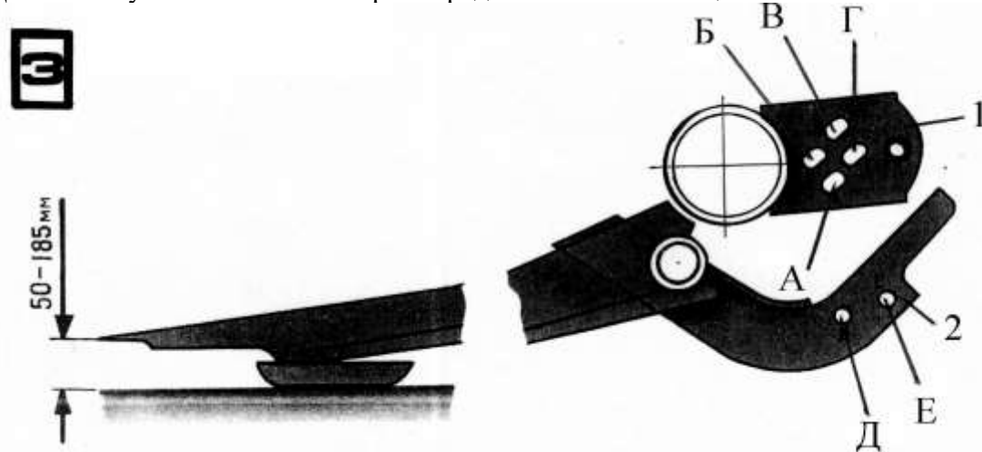
Рис.2.13. Схема регулировки высоты среза: 1 – косынка; 2 – рычаг; А, Б, В, Г, Д, Е – отверстия на рычаге и косынке
