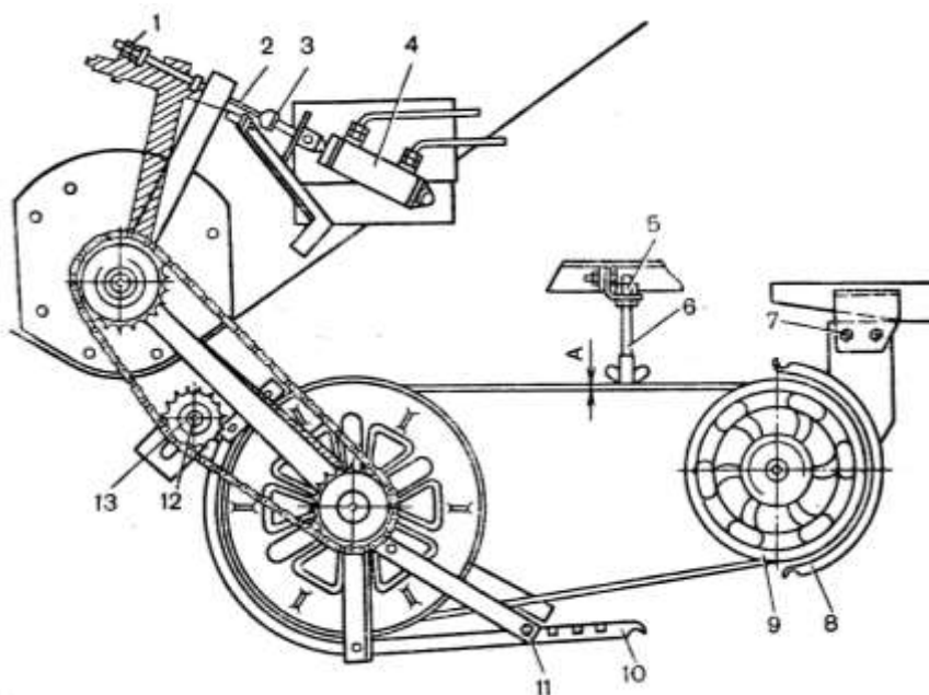
Рис. 7.2. Регулировка механизма включения выгрузного устройства: 1, 3, 5, 7, 11, 12 - гайки; 2 - тяга; 4 - гидроцилиндр; 6 - упор; 8, 10 - щитки; 9 - шкив ведущий; 10 - звездочка натяжная
