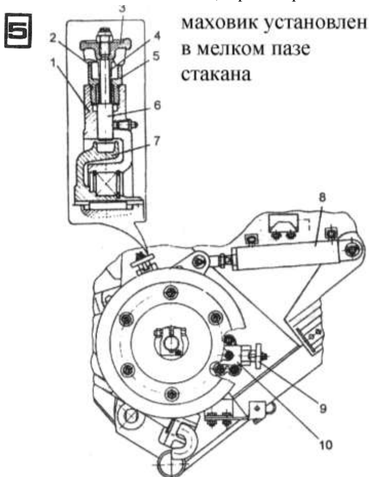
Рис. 3.6. Механизм реверса рабочих органов наклонной камеры: 1 - водило; 2 - мелкий паз стакана; 3, 9 - маховики; 4 - глубокий паз стакана; 5 - стакан; 6 - фиксатор; 7 - храповик; 8 - гидроцилиндр; 10 - кронштейн
