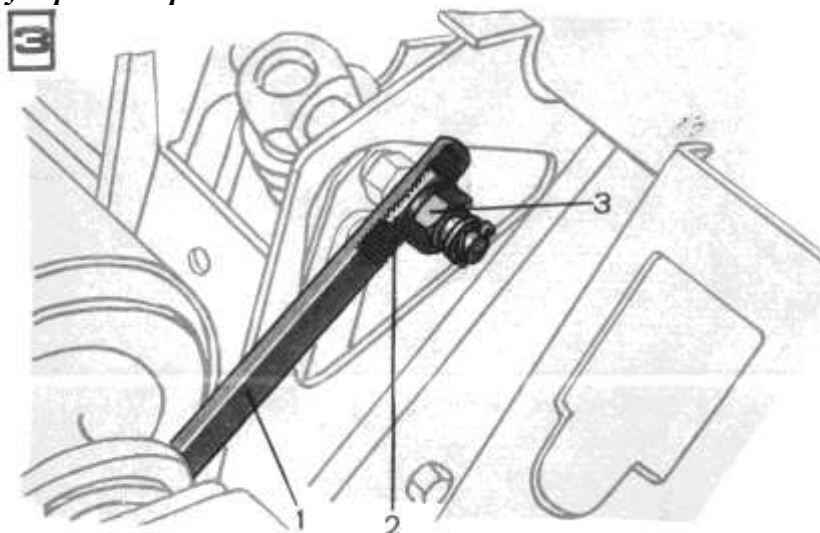
Рис. 5.6 Схема регулировки вертикальности подъемника: 1-тяги; 2-шайба; 3-гайка.
