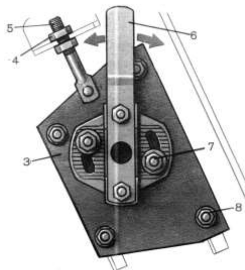
Рис. 2.21. Схема механизма регулировки проставки: 3-плита; 4, 8- гайки; 5-винт; 6-рукоятка; 7-болт
