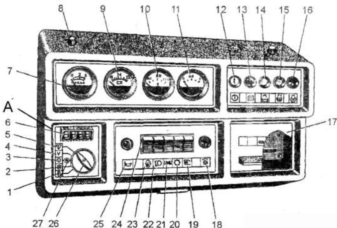
Рис. 15.3. Щиток приборов (см. рис.15.1): 1-контроль оборотов двигателя; 2-обороты вентилятора; 3-обороты барабана; 4- скорость; 5-проверка работы блока; 6-табло; 7- указатель давления масла двигателя; 8-рукоятка съема фальшпанели; 9-вольтметр; 10-указатель температуры воды двигателя или масла ГСТ; 11-указатель уровня топлива; 12-ключ стартера; 13- включатели «массы»; 14-лампа контрольная полного включения леникса выгрузного шнека; 15- включатель магнето-пускового двигателя (СМД-24) или включатель электрофакельного подогревателя (СМД-31А, СМД-23); 16-контроль работы подогревателя; 17-блок предохранителей с переключателем подогревателя в режимы «зима-лето» и розеткой для переноски; 18-сигнализация включения-выключения молотилки; 19-включение автомата сброса копны; 20-включение отопителя; 21-габаритные огни; 22-транспортные фары (в бампере); 23-переключение контроля температуры масла ГСТ и воды двигателя; 24- блок переключателей; 25-звуковой сигнал; 26-переключатель каналов контроля; 27- кнопка запоминания частоты вращения барабана; А-блок измерения частоты вращения (БИЧ)
