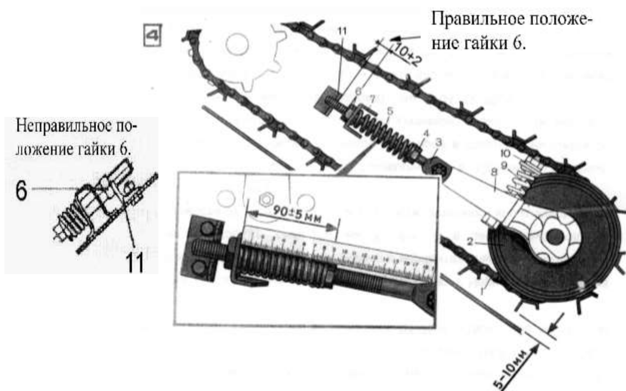
Рис. 3.5. Схема регулировки транспортера: 1 – цепь; 2 – барабан нижний; 3 – винт натяжной; 4,6 – гайка; 5 – пружина; 7 – кронштейн; 8 – опора; 9 – подвеска; 10 – шайба
