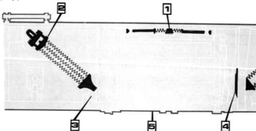
Рис. 2.1. Схема вида жатки сзади (вид сзади): 1 – растяжки; 2 – блоки пружин; 3 – механизм подвески левый; 4 – боковые щитки; 5 – переходной щиток
