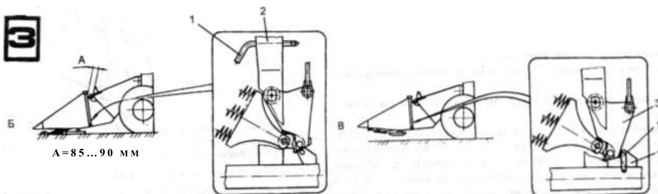
Рис. 2.4. Положение механизма уравнивания при работе жатки: Б - при работе с копированием рельефа поля: жатка опирается на башмаки, штыри 1 установлены в стойках 2 корпуса, зазор А равен 85...90 мм; В - при работе без копирования рельефа поля или при транспортировании на небольшие расстояния с поднятой жаткой: штыри 1 установлены в отверстиях кронштейнов 4, рычаги 3 опираются на штыри
