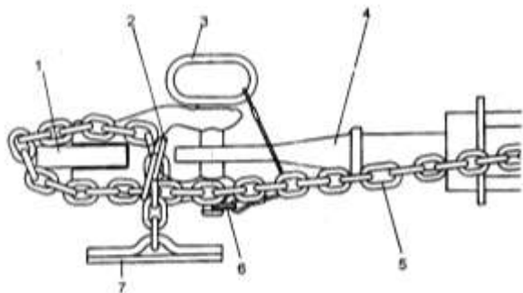
Рис. 24.4. Сцепка тележки с комбайном или трактором: 1-поперечина прицепного устройства трактора; 2-петля специальная цепи; 3-шкворень; 4-петля специальная тележки; 5-цепь; 6-шплинт быстроразъемный; 7-штырь цепи
