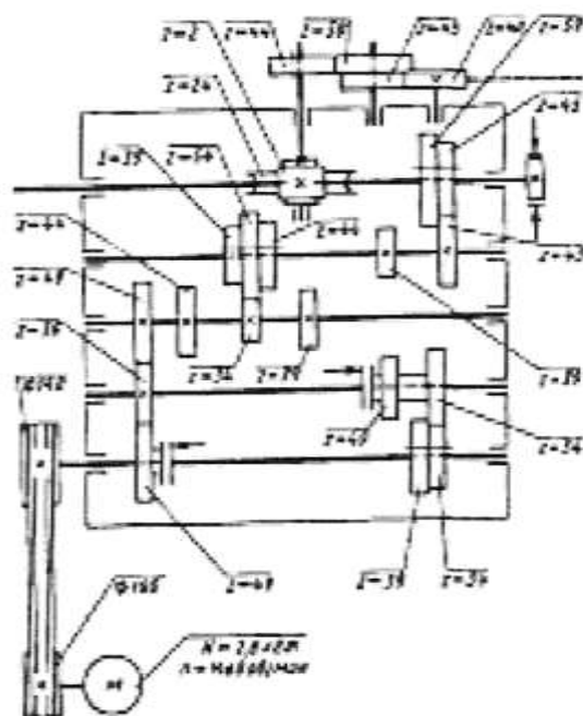
Кинематическая схема коробки скоростей токарно-револьверного станка П326
