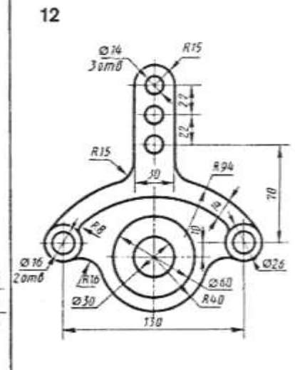
Подвеска
