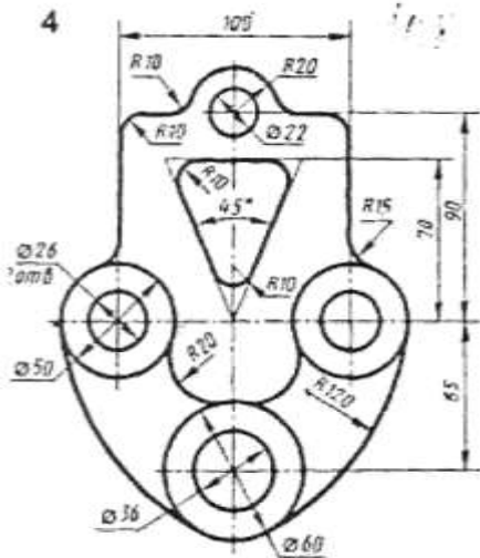
Подвеска
