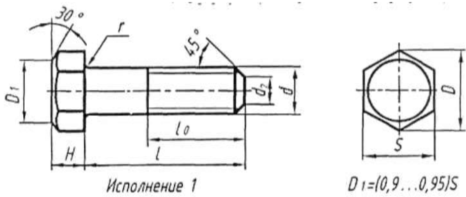
Рис. Болт
