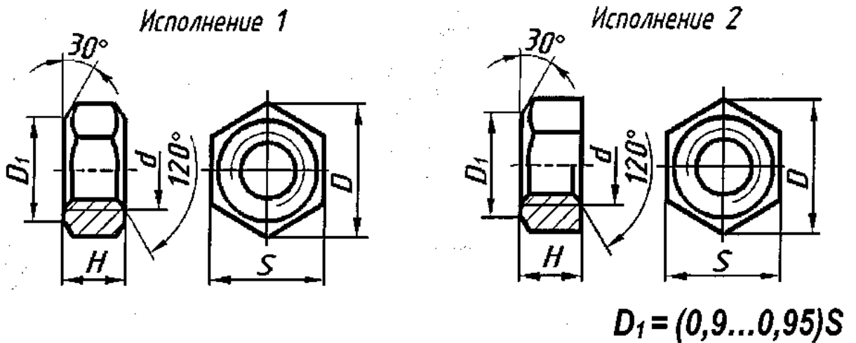
Рис. Гайка в двух исполнениях
