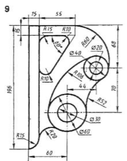
Кронштейн
