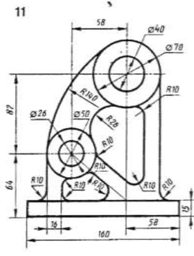
Станина
