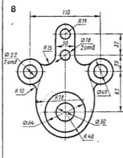
Подвеска
