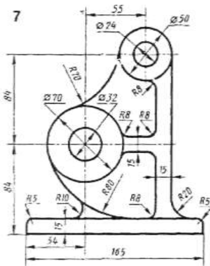
Станина
