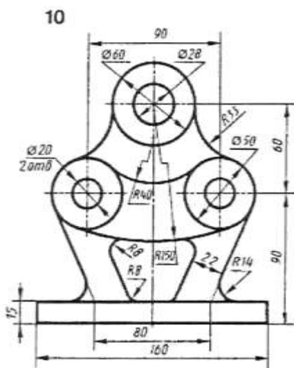
Станина
