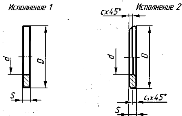
Рис. Шайба в двух исполнениях
