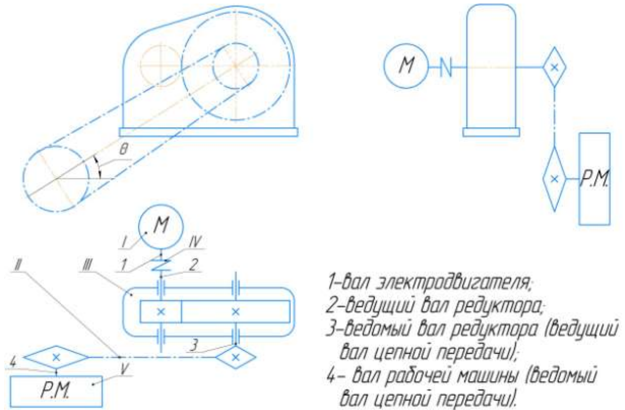
Рисунок 12 – Кинематическая схема привода: I – электродвигатель; II – цепная передача; III – цилиндрический редуктор; IV – муфта соединительная; V – рабочая машина
