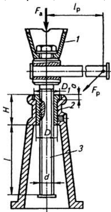
Рисунок 5.3.1 – Схема винтового домкрата:
