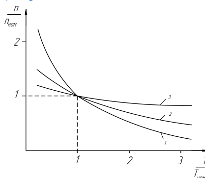
Рисунок 3.1.1 – Механические характеристики двигателей постоянного тока
