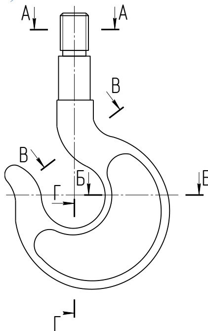
Рисунок 2.1.1 – Схемы опасных сечений грузового однорогого крюка.
