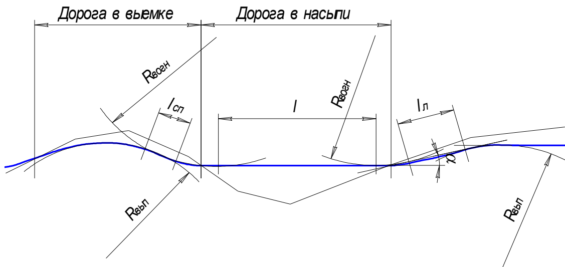
Рисунок 2.18 – Схематическое изображение продольного профиля дороги
