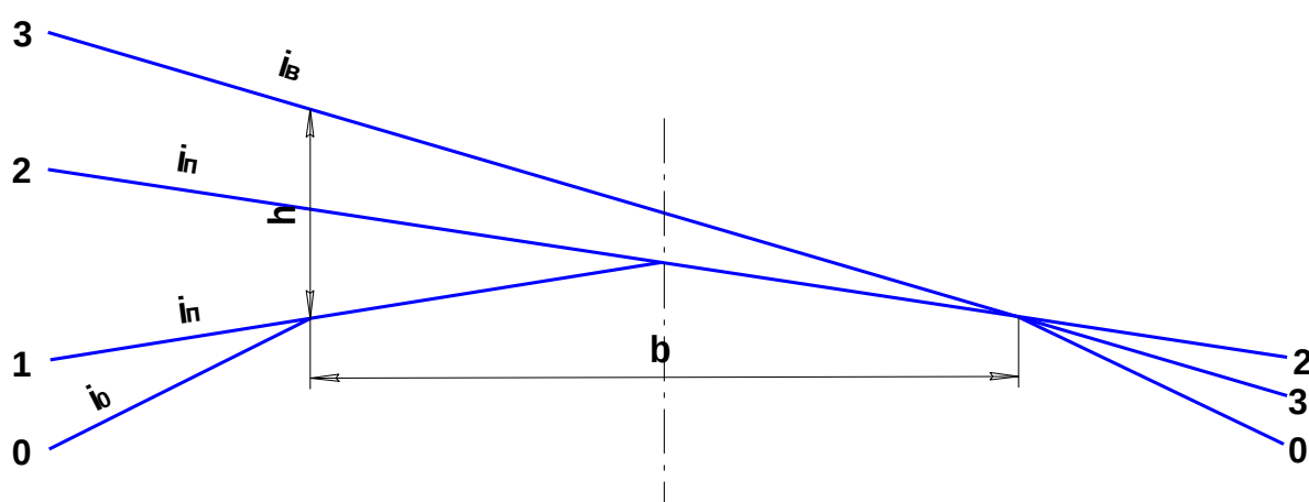
Рисунок 2.12 – Последовательность изменения поперечного профиля на обгоне виража
