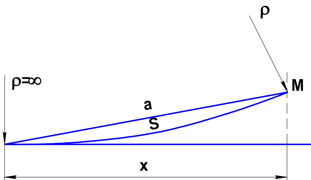
Рисунок 2.8 – Элементы переходных кривых
