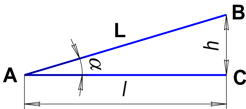
Рисунок 2.19 – Определение продольного уклона дороги
