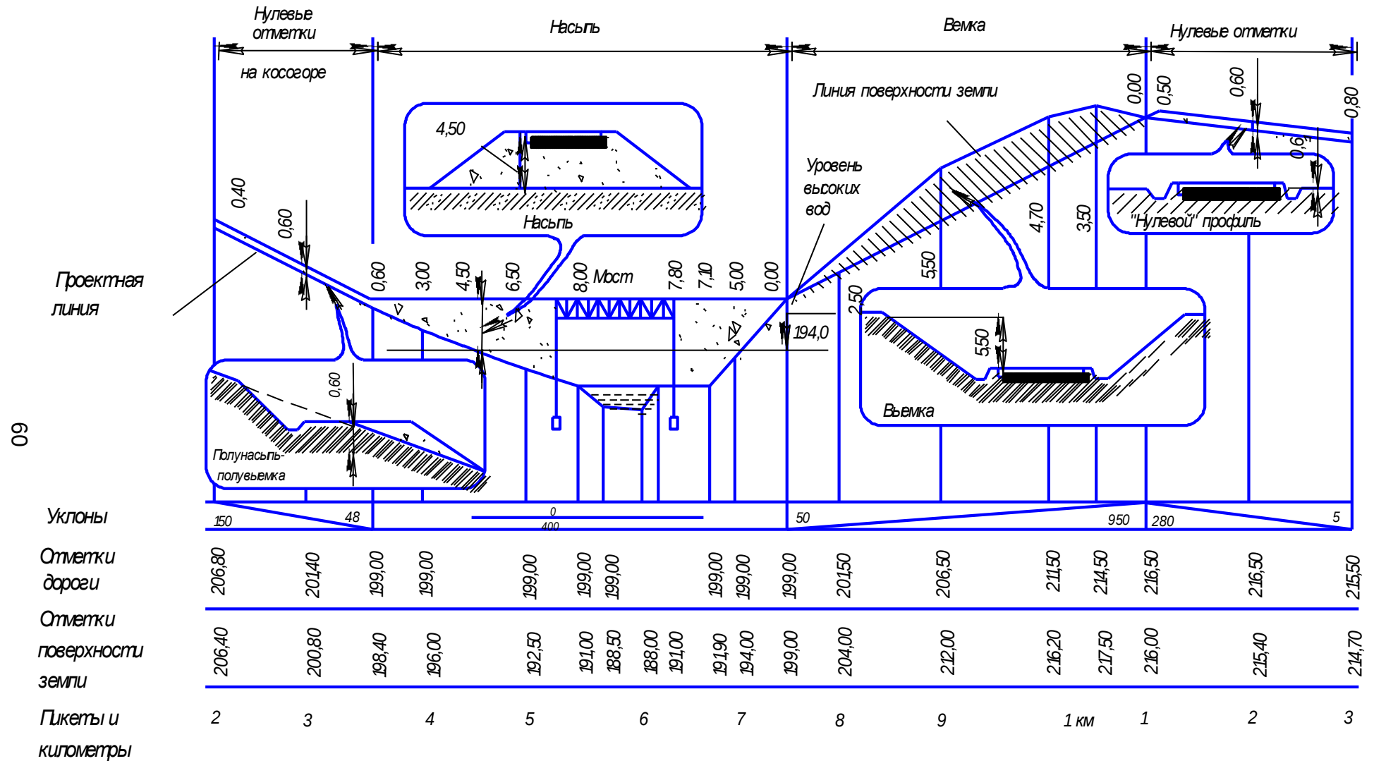
Рисунок 2.17 – Продольный профиль автомобильной дороги
