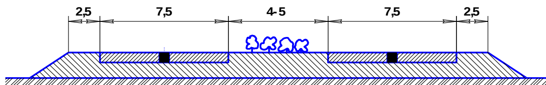
Рисунок 2.4 – Автомобильная дорога с разделительной полосой
