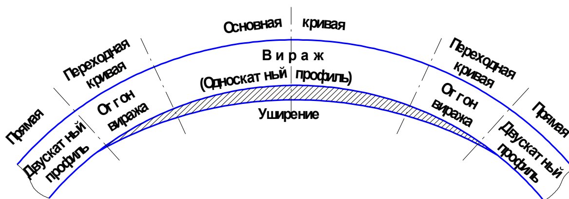
Рисунок 2.13 – План проезжей части на закруглении с виражом
