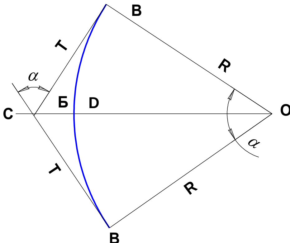
Рисунок 2.22 – Элементы кривой
