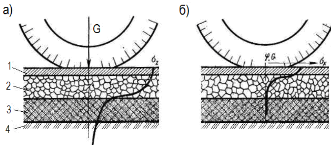
Рисунок 2.25 – Распределение напряжений в дорожной одежде от колес автомобилей: а – эпюра вертикальных напряжений; б – эпюра горизонтальных напряжений; 1 – покрытие; 2 – основание; 3 – дополнительный слой основания; 4 – грунт земляного полотна
