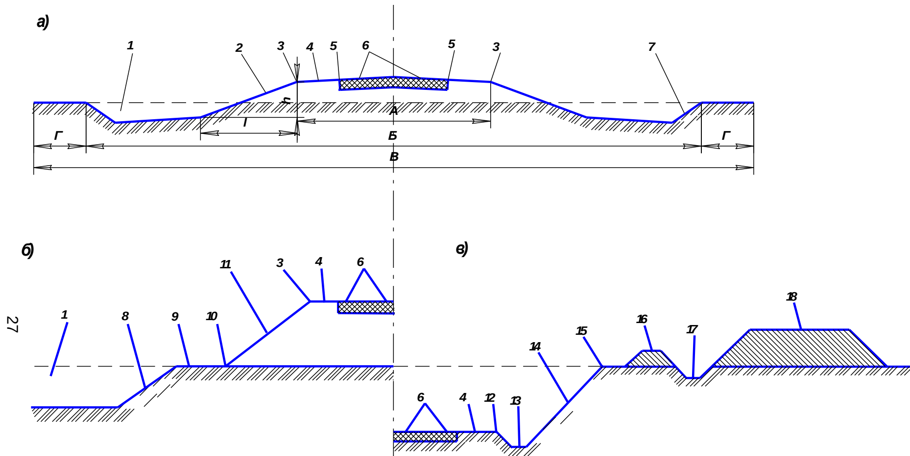
Рисунок 2.1 – Основные элементы дороги в поперечном профиле:
